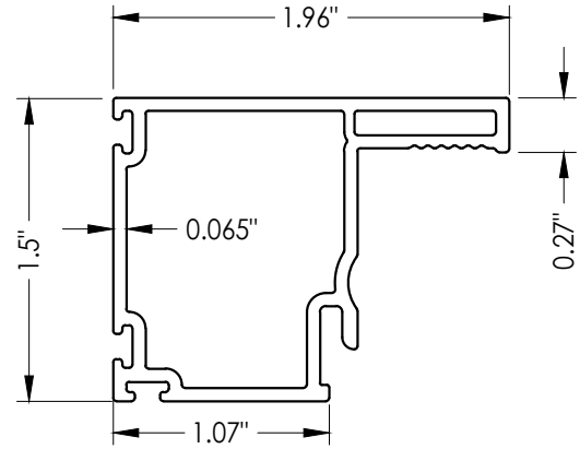
8 PLAIN STILE
